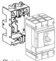
Plug-in Configuratio
